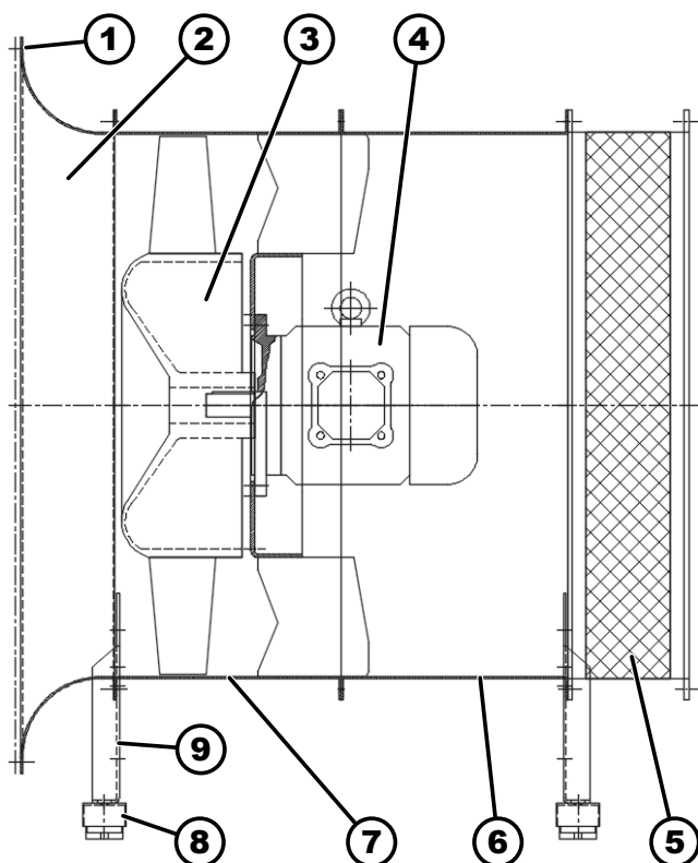
Abb. 47: Übersicht Ersatzteile
