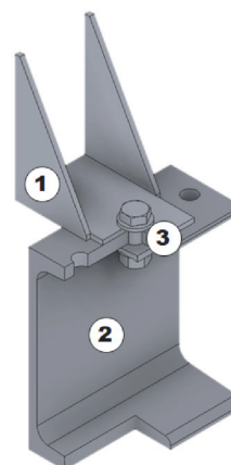
Abb. 37: Verbindung Pratze Stahlbau/Schiene
