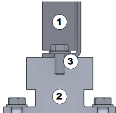
Abb. 32: Verbindung Schachtfuß/Schwingungsdämpfer
