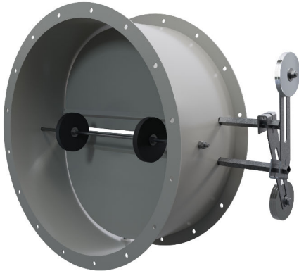
Abb. 16: Selbsttätige Verschlussklappe
