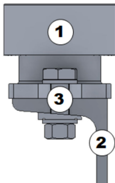
Abb. 34: Verbindung Schwingungsdämpfer/Stahlbau/Schiene
