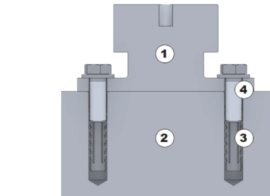
Abb. 33: Verbindung Schwingungsdämpfer/Boden
