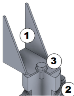
Abb. 36: Verbindung Pratze/Schwingungsdämpfer
