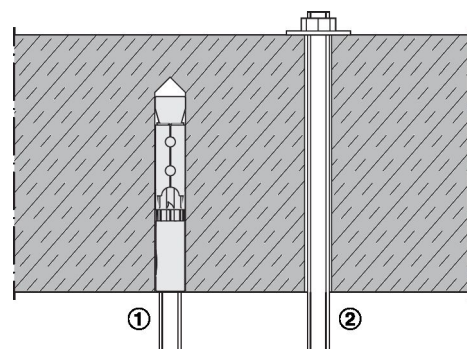
Abb. 41: Deckenbefestigung
